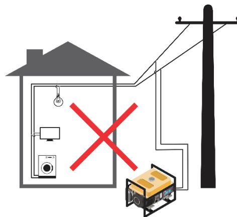
Fig.7 – Ligação direta na rede
