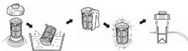
Fig. 12 – Filtro de Combustível
