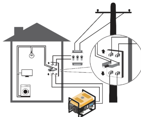
Fig. 8 – Ligação com chave de transferência
