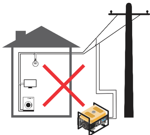
Fig.8 – Ligação direta na rede
