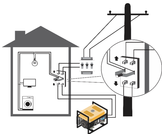
Fig. 9 – Ligação com chave de transferência
