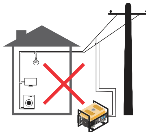
Fig.8 – Ligação direta na rede
