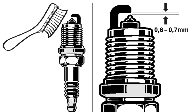
Fig. 13 – Vela de Ignição
