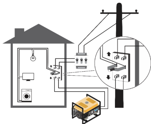
Fig. 11 – Ligação com chave de transferência
