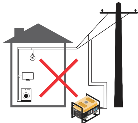
Fig.10 – Ligação direta na rede
