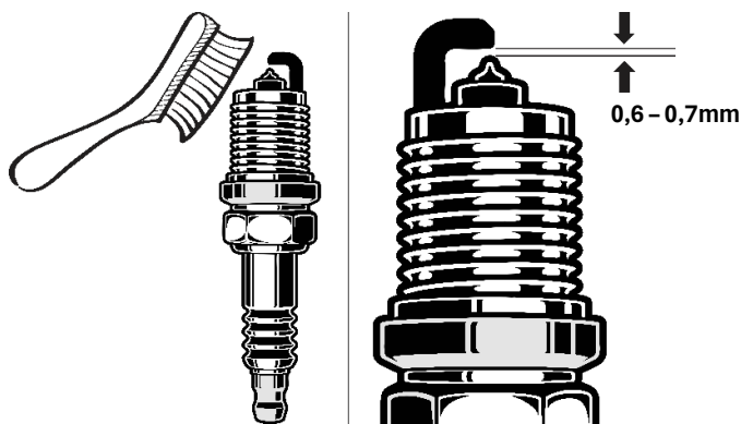
Fig. 11 – Vela de Ignição
