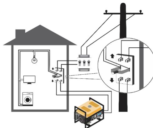
Fig. 9 – Ligação com chave de transferência
