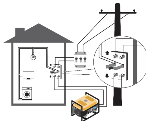
Fig. 10 – Ligação com chave de transferência
