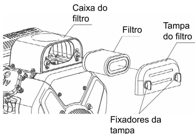
Fig.13 – Troca do filtro
