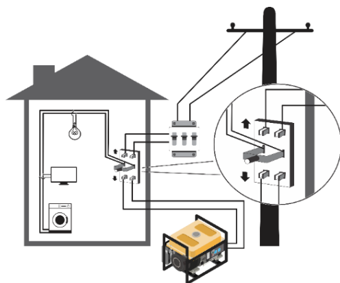
Fig. 12 – Ligação com chave de transferência
