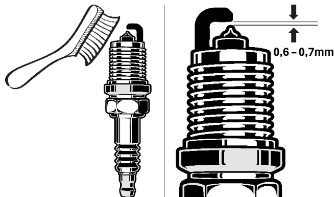
Fig. 10 – Vela de Ignição
