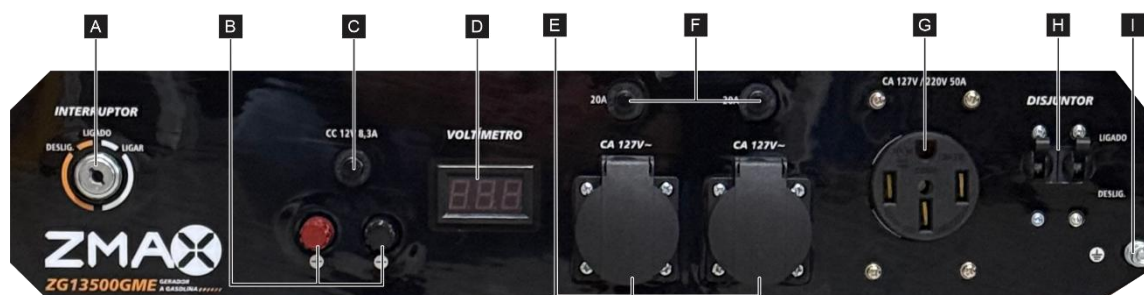
Fig. 4 – Painel de controle
