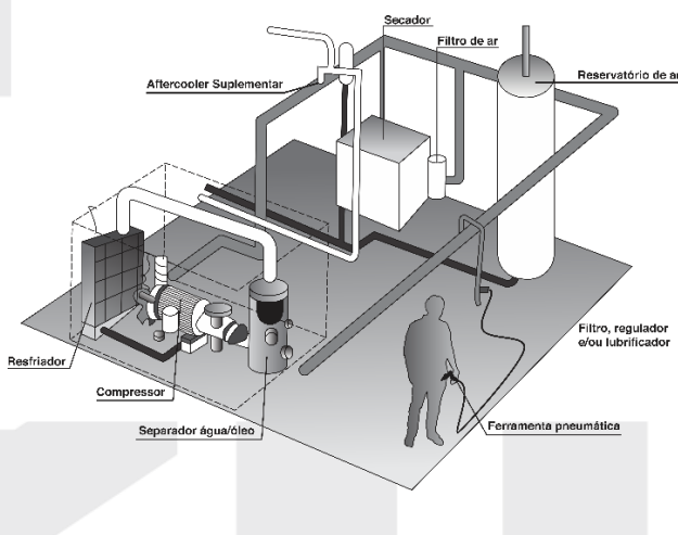
Fig. 3 – Rede de ar comprimido industrial
