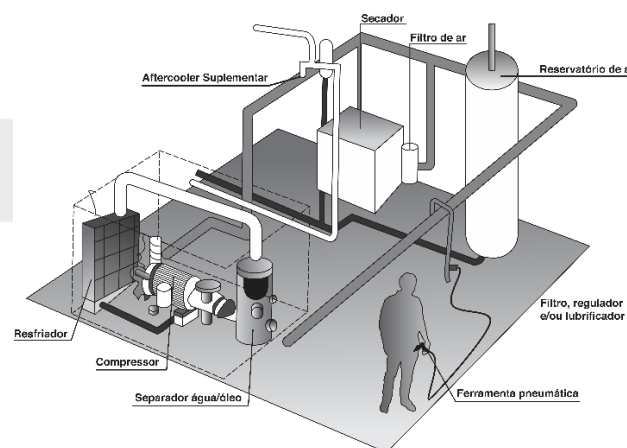
Fig. 3 – Rede de Ar comprimido industrial
