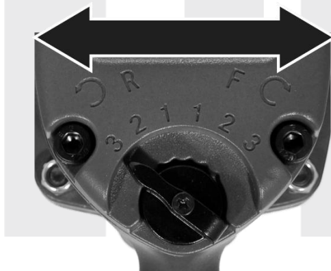
Fig. 15 - Sentido de rotação
