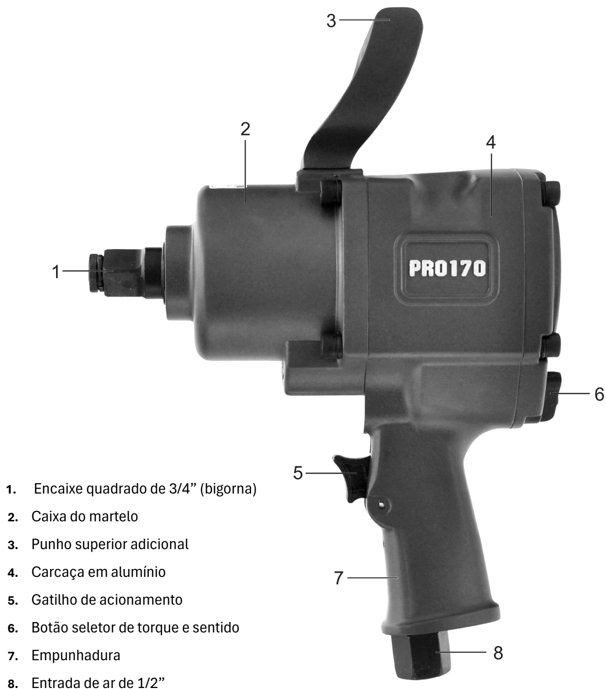
Fig. 4 – Componentes simplificados
