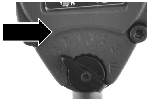
Fig. 16 - Níveis de torque (aperto)
