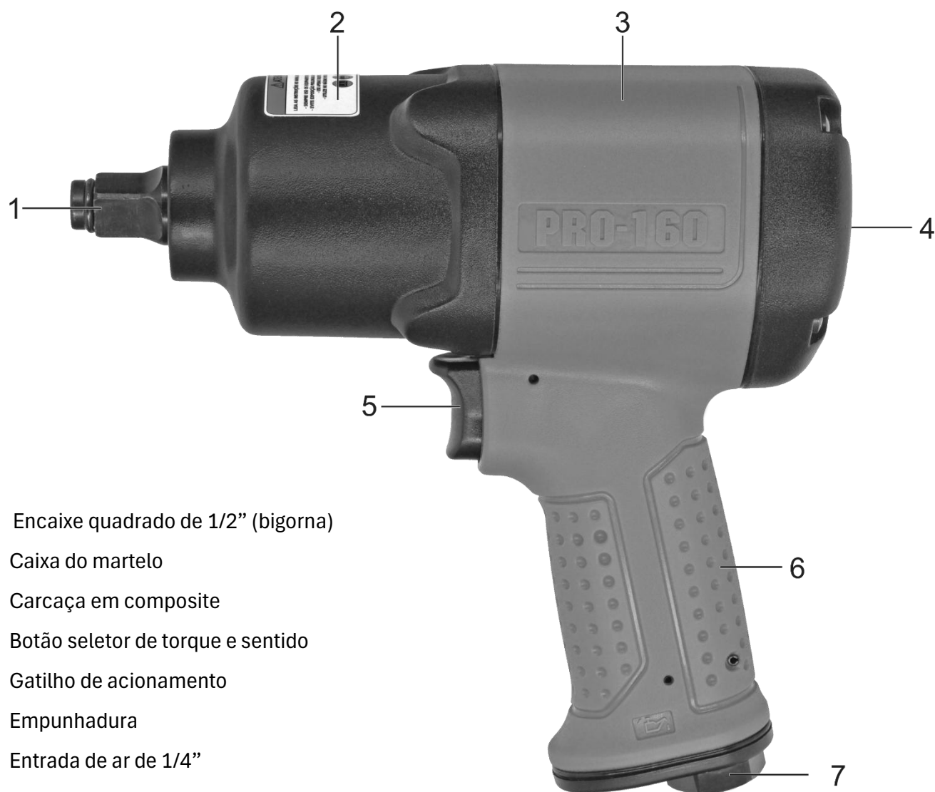
Fig. 4 – Componentes simplificados
