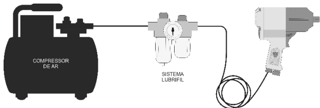
Fig. 1 – Requisitos pneumáticos
