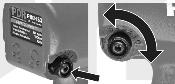
Fig. 17 – Níveis de torque (desaperto)
