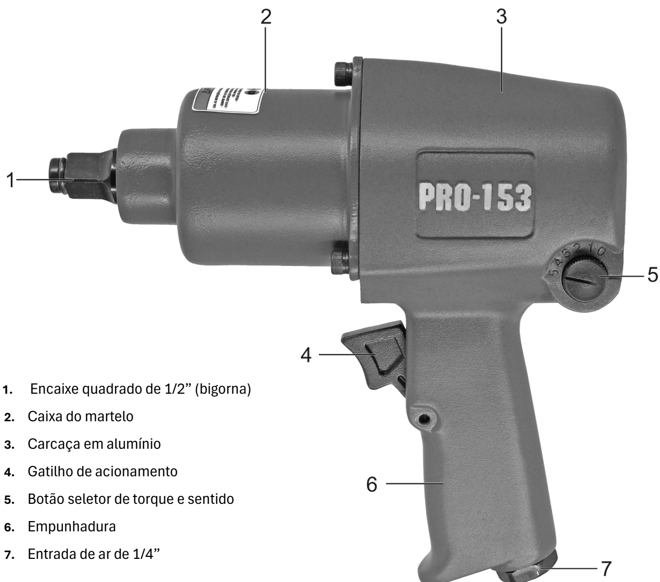
Fig. 4 – Componentes simplificados
