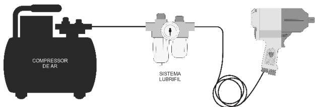
Fig. 1 – Requisitos pneumáticos
