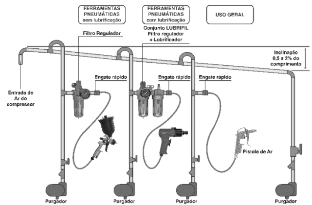
Fig. 2 – Rede de Ar comprimido padrão
