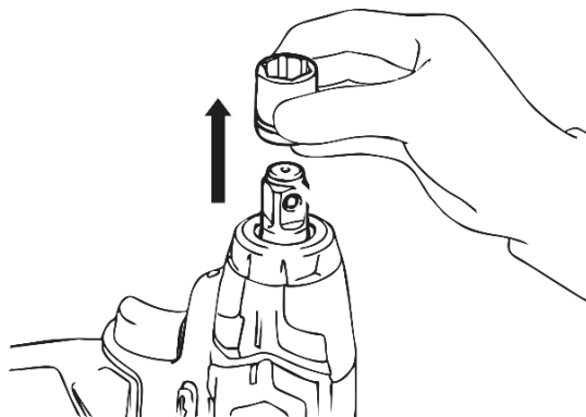
Fig. 6 – Retirada do soquete
