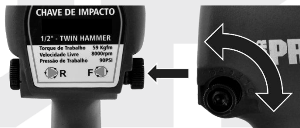
Fig.17 - Níveis de torque (desaperto)
