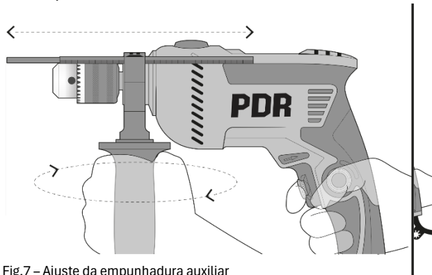
Fig.7 – Ajuste da empunhadura auxiliar
