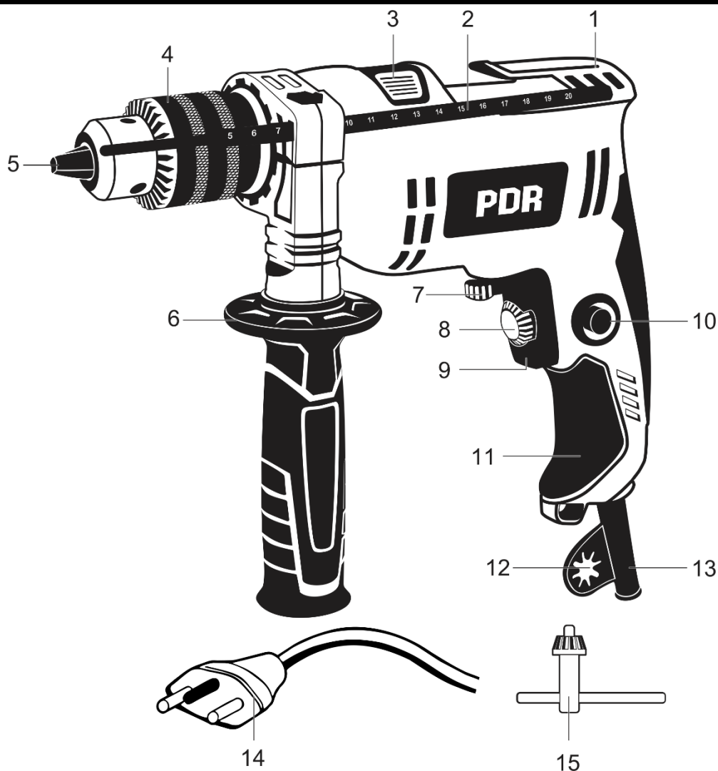
Fig. 1 – Componentes simplificados
