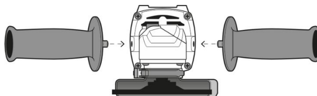
Fig. 2 – Montagem da empunhadura auxiliar
