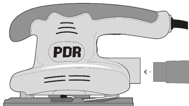
Fig.10 – Instalação do aspirador de pó
