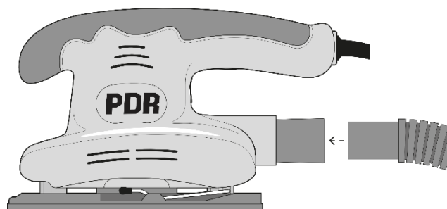
Fig.11 – Instalação do aspirador de pó
