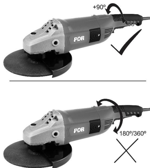
Fig. 3 – Cabo giratório
