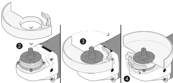
Fig. 4 – Montagem da capa de proteção
