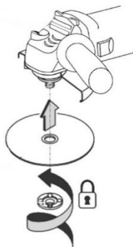
Fig. 10 – Troca do disco
