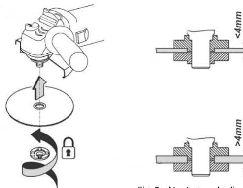
Fig. 6 – Montagem do disco
