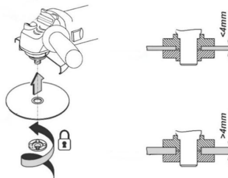
Fig. 6 – Montagem do disco
