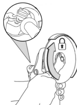
Fig. 7 – Montagem do disco
