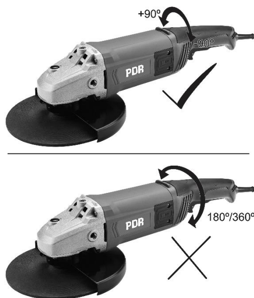
Fig. 3 – Cabo giratório
