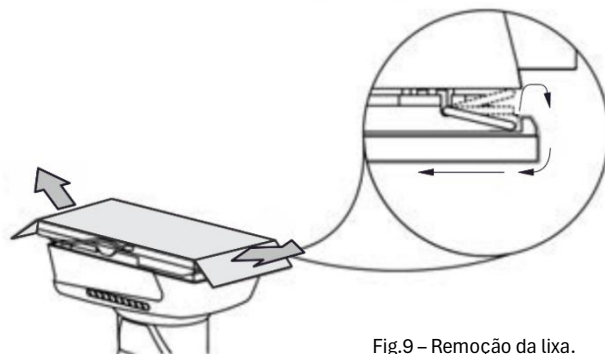
Fig.9 – Remoção da lixa.
