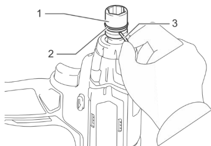
1 – Soquete de impacto 2 – O-ring 3 – Pino
