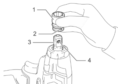
1 - Soquete de impacto 2 - Buraco 3 - Eixo quadrado 4 - Pino de retenção
