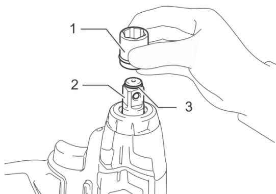
1 – Soquete de impacto 2 – Acionamento quadrado 1/2 3 – Mola do anel
