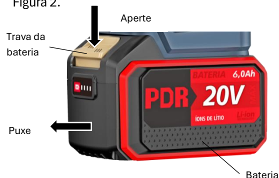
Fig. 2 – Retirando a bateria
