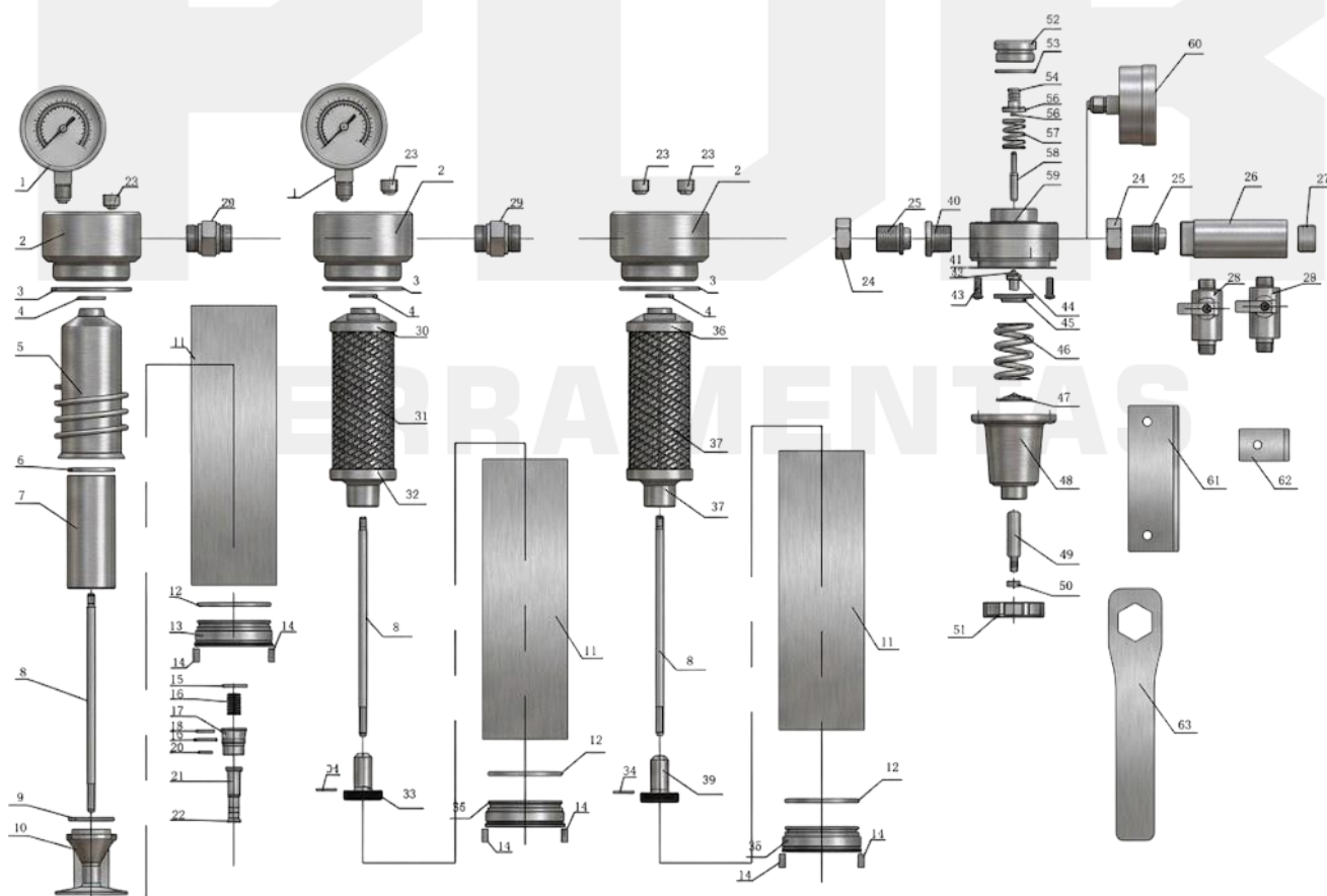
Fig. 3 - visão geral - vista explodida
