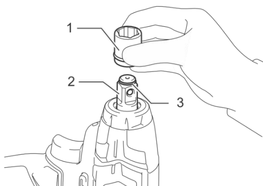
Fig. 3 – Encaixe 1/2" Quadrado (1)
