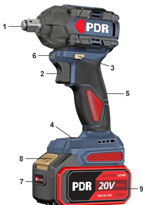
Fig. 1 – Componentes
